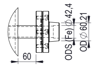
DETTAGLIO B SCALA 2 : 15
